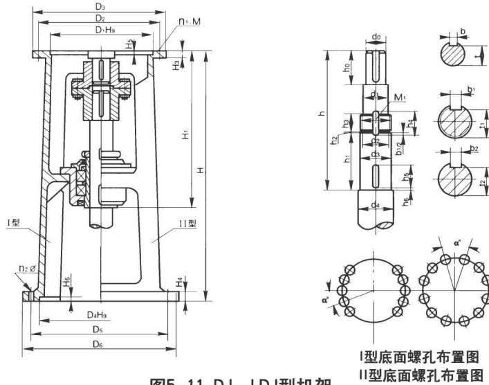
图5-11 DJ、LDJ型机架
