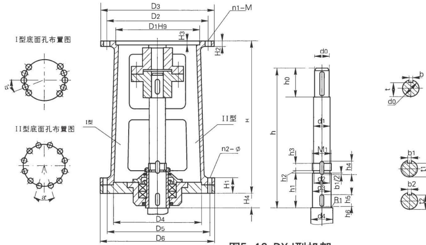
图5-12 DXJ型机架
