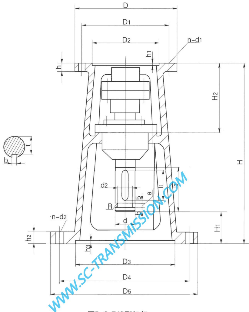
图5-6 TJQ型机架
